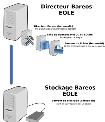
Architecture de Bareos intégré à EOLE
