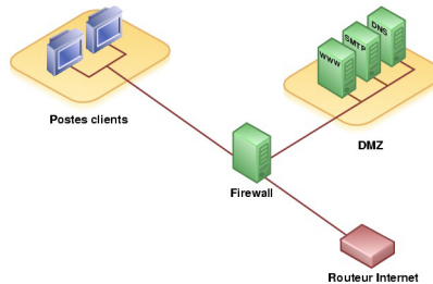
Diagramme d'une DMZ
