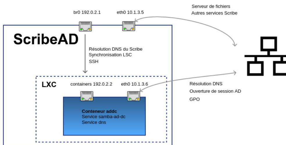
Les flux réseaux entre le conteneur et le maître
